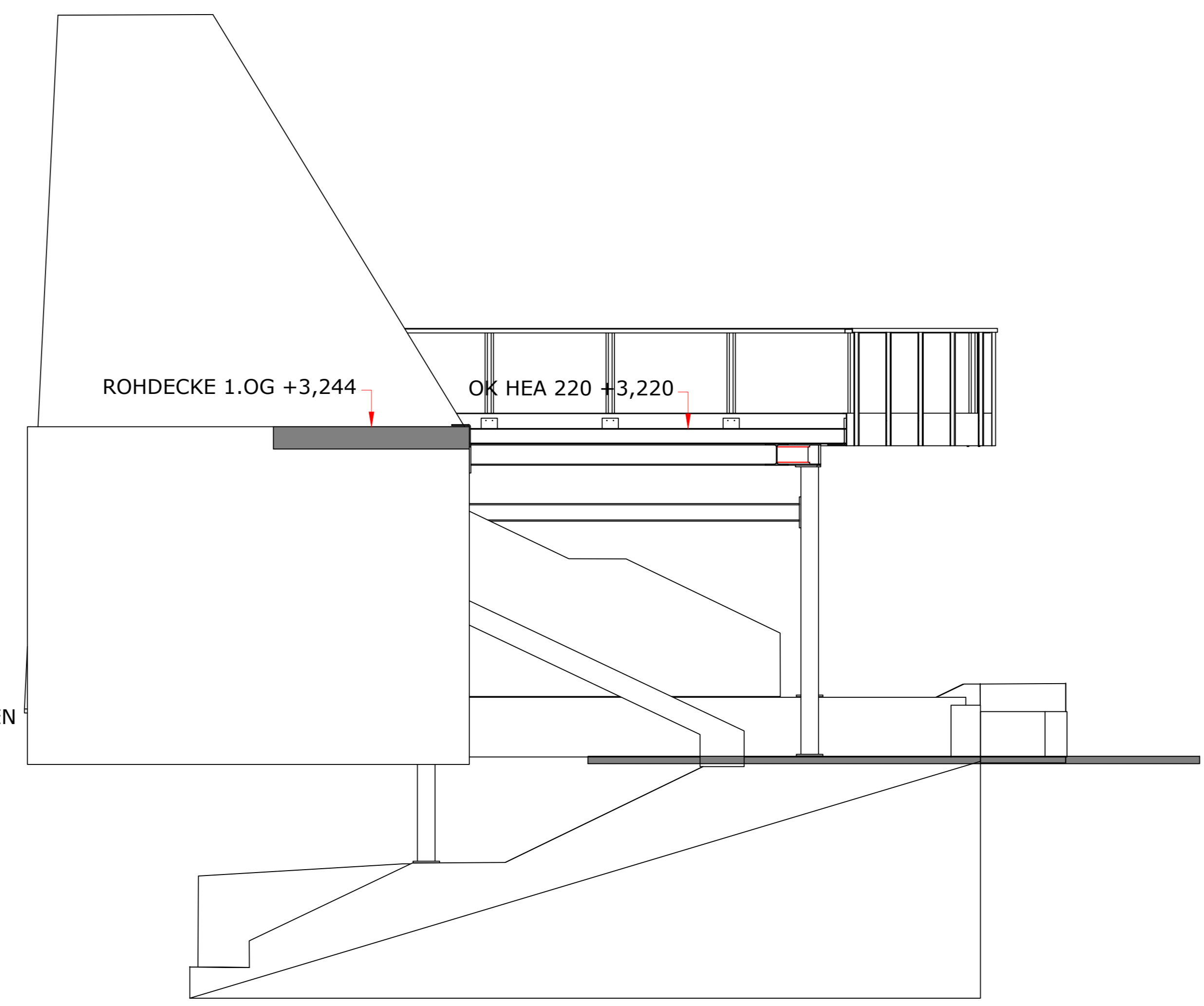
Schnitt 2-2
