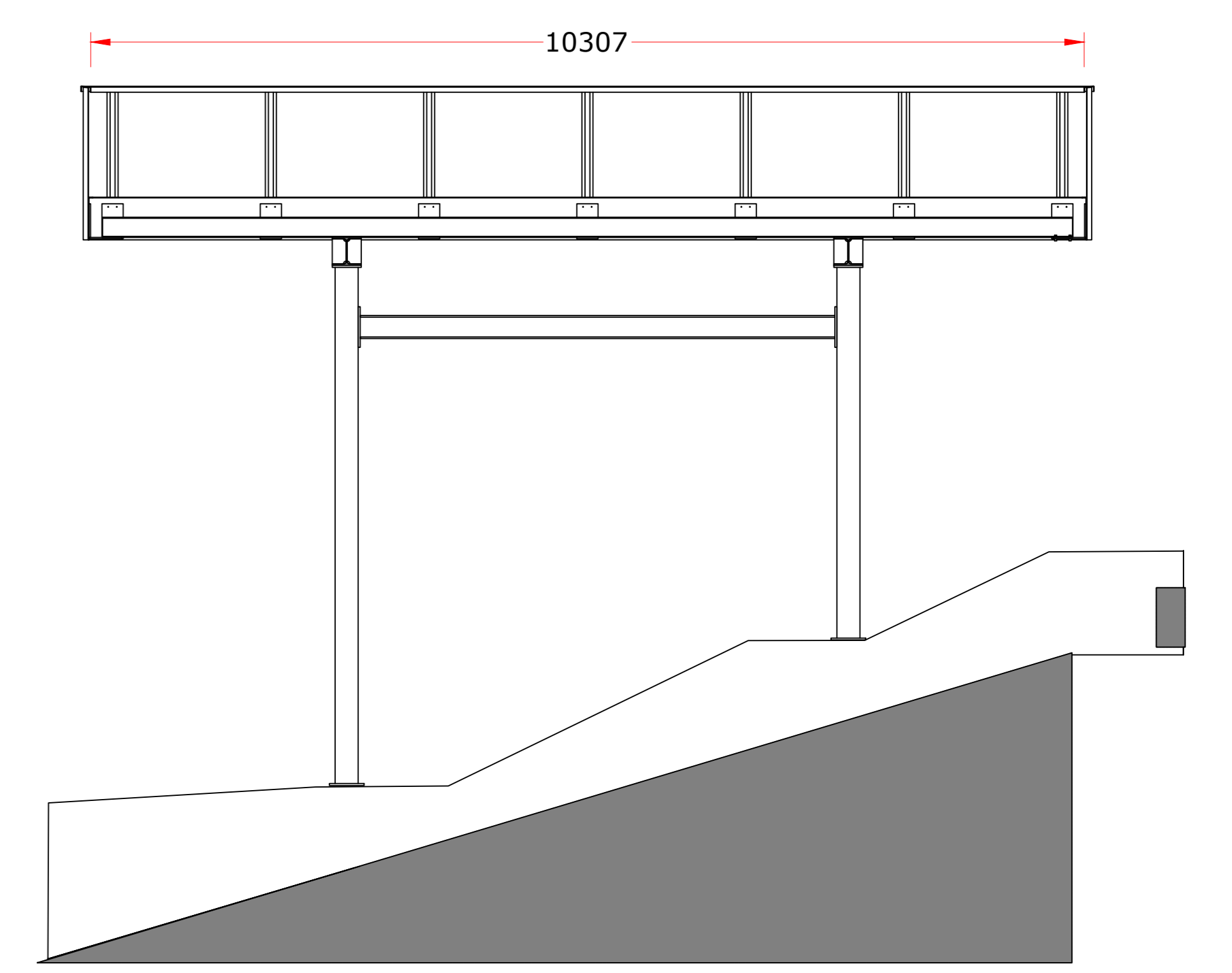
Schnitt 1-1
