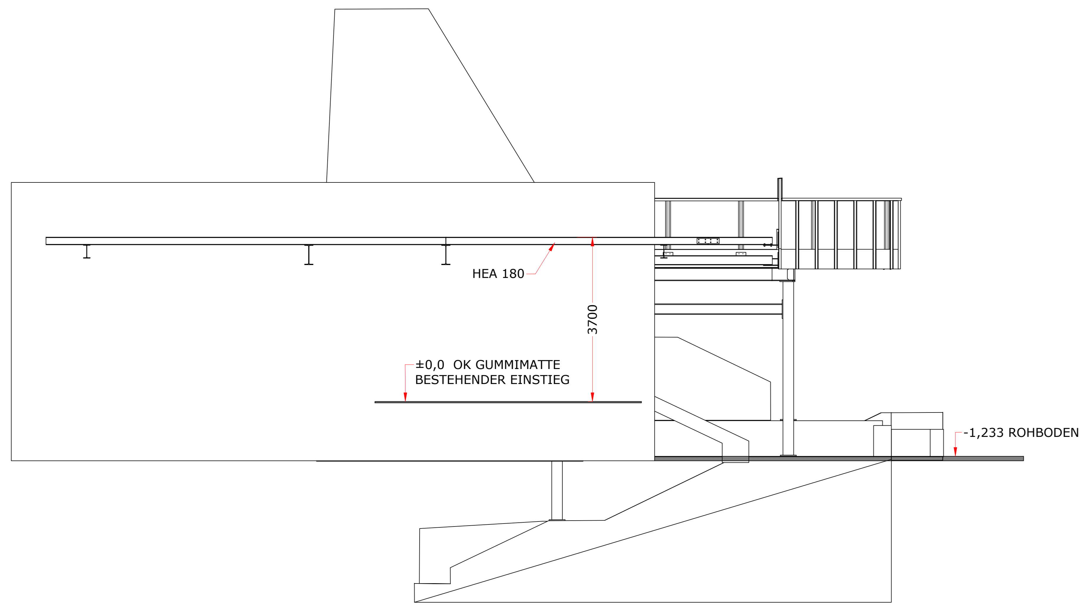
Schnitt 3-3
